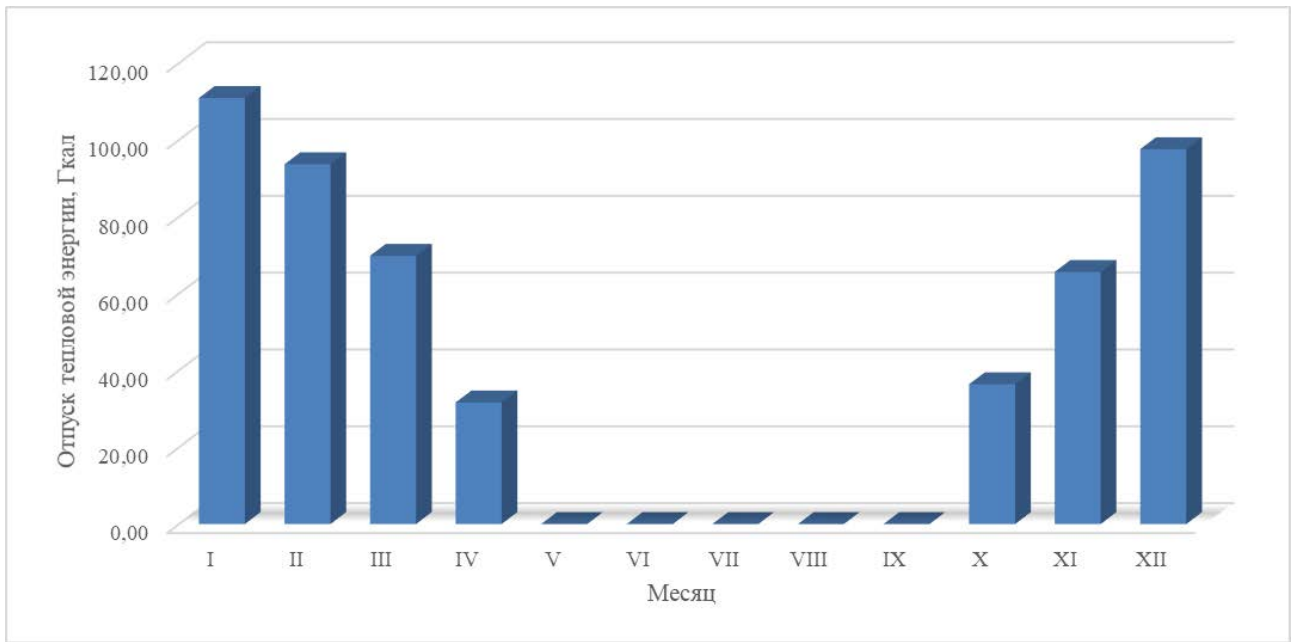
Рисунок 1.3 – Оптимальный температурный график отпуска тепловой энергии по сельской котельной
